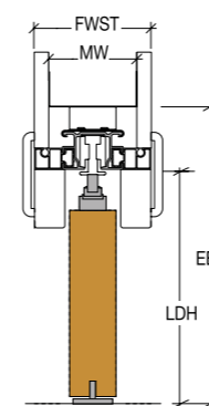
Vertikaler Querschnitt
