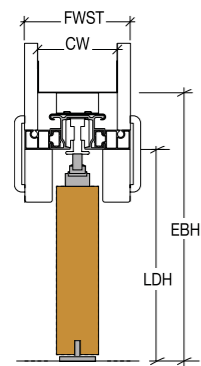
Vertikaler Querschnitt
