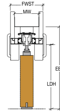
Vertikaler Querschnitt
