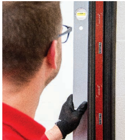
10 Ausrichten, anklopfen, fertig!
