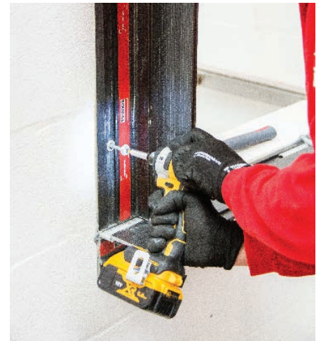
11 Rahmendübel anbringen und einschrauben
