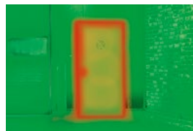
Sichtbarer Energieverlust ohne thermisch getrennte Tür
