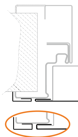
Eck-/Gegenzarge (Dünn-/Dickfalztür)
