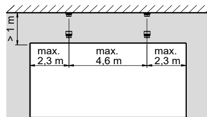
Fall 5: Öffnungsbreite > 4,6 m und \leq 8 m Sturzhöhe einseitig oder beidseitig > 1 m. 6 Stück Rauchmelder, davon 4 Stück an der Decke und 2 Stück vor dem Sturz montiert.
