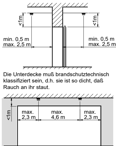
Fall 2: Öffnungsbreite > 4,6 m und \leq 8 m Sturzhöhe beidseitig < 1 m. 4 Stück Rauchmelder an der Decke montiert.
