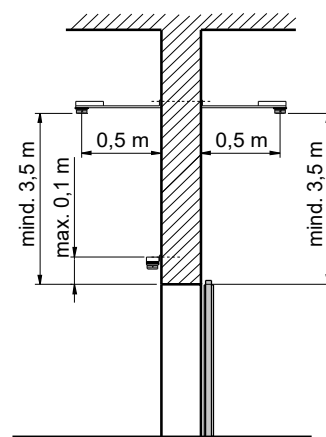
Fall 3: Öffnungsbreite > 8 m Sturzhöhe beidseitig < 1 m. 6 Stück Rauchmelder an der Decke montiert.
