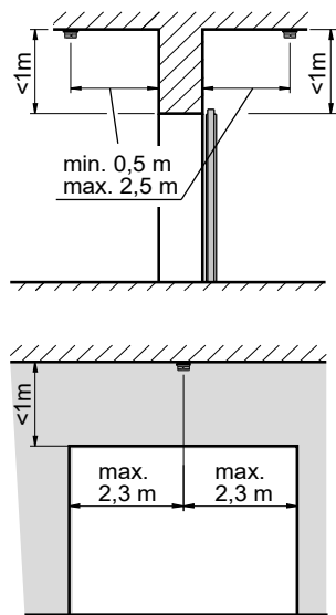
Fall 1: Öffnungsbreite \leq 4,6 m und Sturzhöhe beidseitig < 1 m. 2 Stück Rauchmelder an der Decke montiert.
