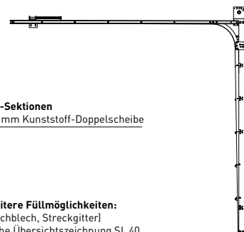
Normal-Beschlag
