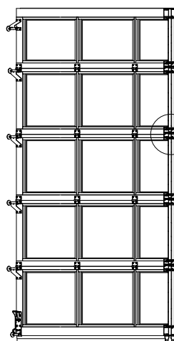
Schnitt Torblatt
