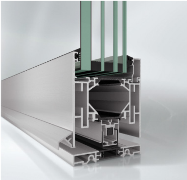
Schüco FireStop ADS 90 FR 30-CE (0 mm Schwelle)
