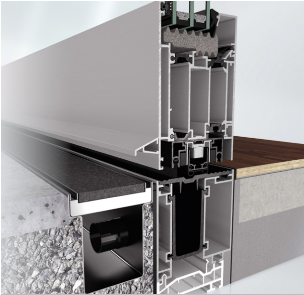
Schüco AD UD 75 mit barrierefreier Nullschwelle und Entwässerung
