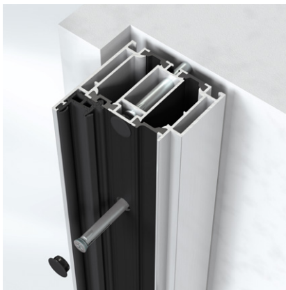
Symmetrischer Profilaufbau für system- und bautiefen-übergreifende identische Fertigungsprinzipien
