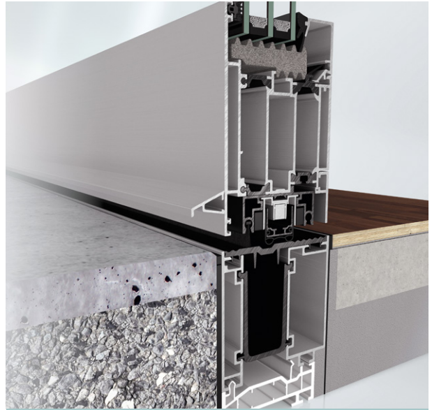
Schüco AD UD 75 mit barrierefreier Nullschwelle
