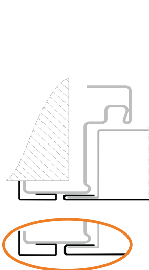
Eckzarge (Dünn-/Dickfalztür)
