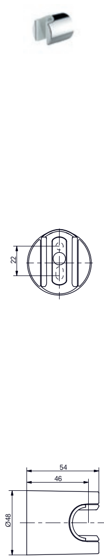
Brausehalter mit Verdrehenschutz Shower hook with anti-rotation protection
