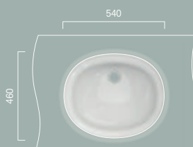
LW764Y Unterbauwaschtisch rund 540 mm ohne Hahnloch, mit Überlauf Undercounter basin round 540 mm without tap hole, with overflow
