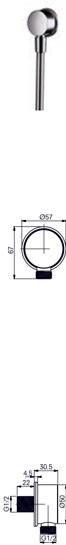
Wandanschlussbogen 1/2" Shower elbow 1/2"
