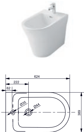
Bidet MH, bodenstehend mit Hahnloch, mit Überlauf Bidet MH, floor-standing with tap hole, with overflow
