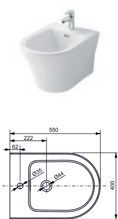
Bidet MH, wandhängend mit Hahnloch, mit Überlauf Bidet MH, wall-hung with tap hole, with overflow
