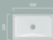
MRZ710BCB1 LUMINIST/S Aufsatzwaschtisch 500 mm LUMINIST/S vessel 500 mm
