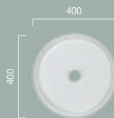
MRZ700BCB1 LUMINIST/R Aufsatzwaschtisch 400 mm LUMINIST/R vessel 400 mm
