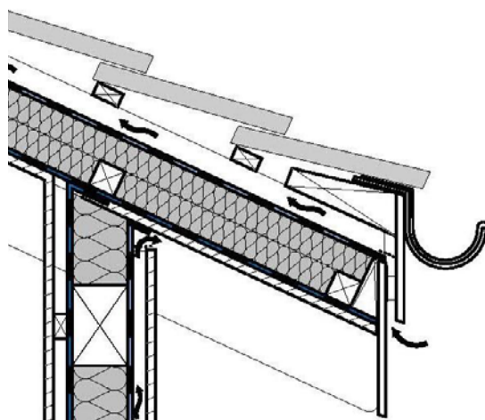
Traufanschluss
