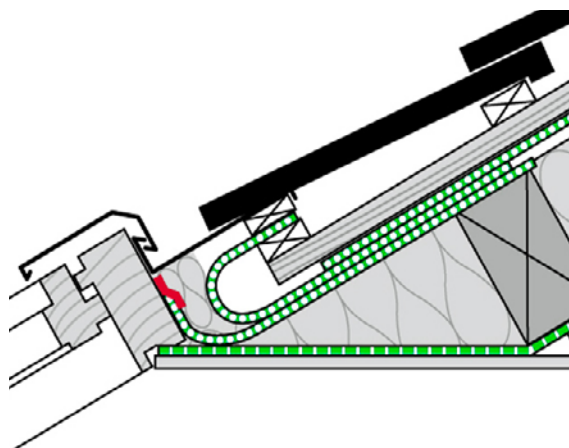
Fensteranschluss
