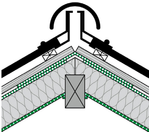
Firstanschluss
