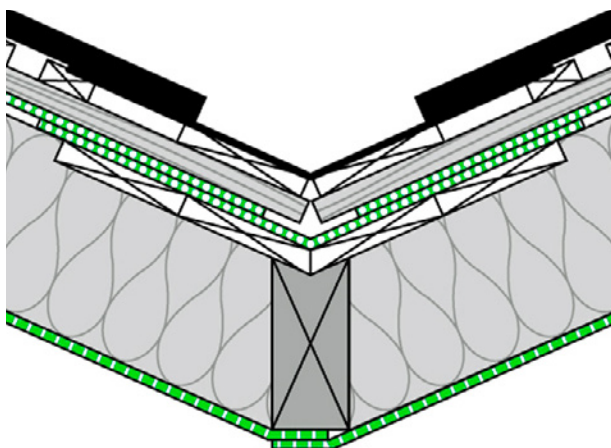
Verklebung Kehle
