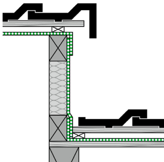
Gaubenanschluss
