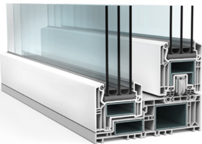
Die Designvariante VEKAMOTION 82 MAX steigert den Glasanteil mit ihrem besonders schlanken Festflügel nochmals deutlich
