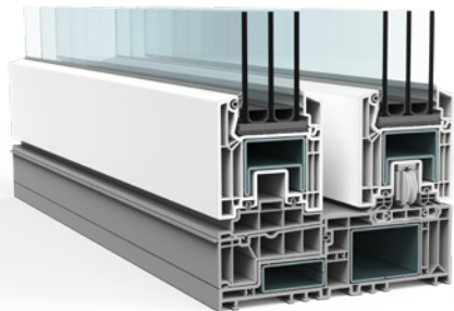
VEKAMOTION 82 bietet schon in der Grundvariante einen hohen Glasanteil mit lediglich 86 mm Flügelhöhe
