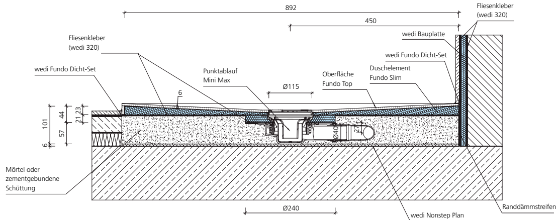
wedi Fundo Punktablauf Mini Max, DN 40, auf Estrichfußboden
