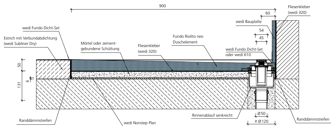
wedi Fundo Rinnenablauf senkrecht, DN 50, Estrichfußboden
