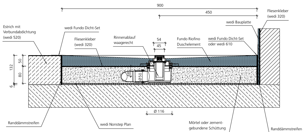
wedi Fundo Rinnenablauf waagrecht, DN 50, Estrichfußboden
