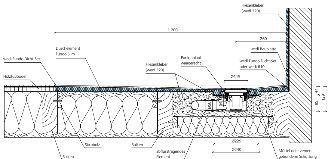
wedi Fundo Punktablauf waagerecht, DN 50, in Holzbalkendecke
