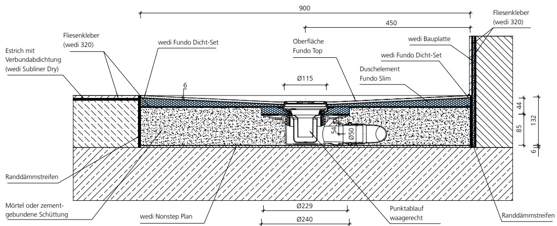
wedi Fundo Punktablauf waagerecht, DN 50, in Estrichfußboden
