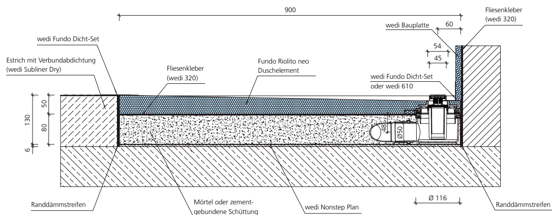
wedi Fundo Rinnenablauf waagrecht, DN 50, Estrichfußboden
