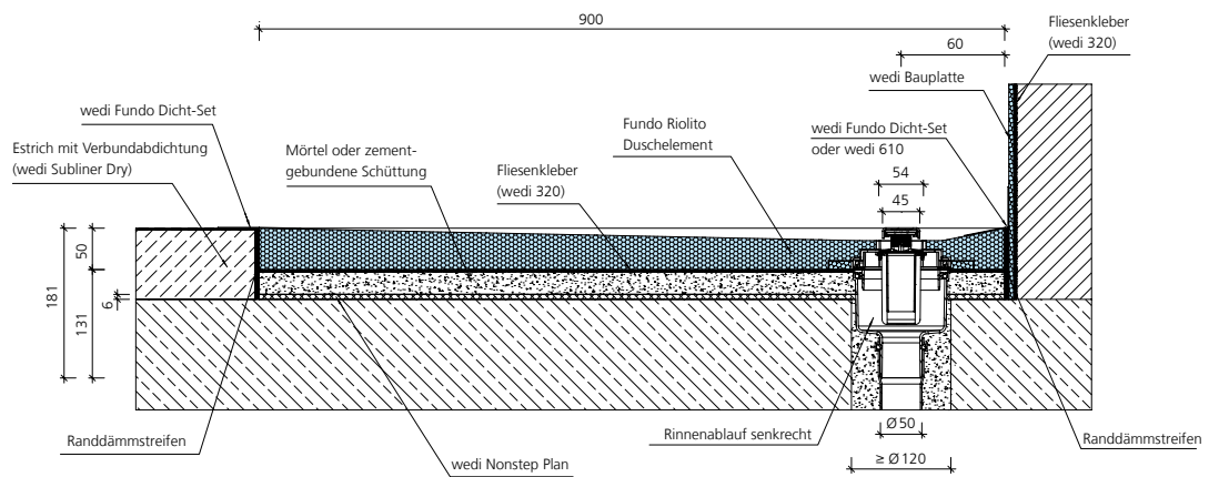
wedi Fundo Rinnenablauf senkrecht, DN 50, Estrichfußboden
