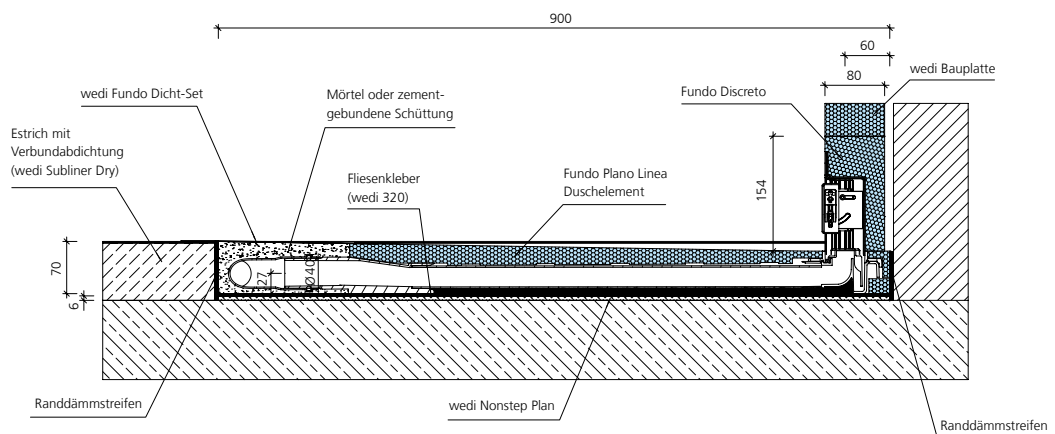
Fundo Discreto, Wandablauf, DN 40, Estrichfußboden
