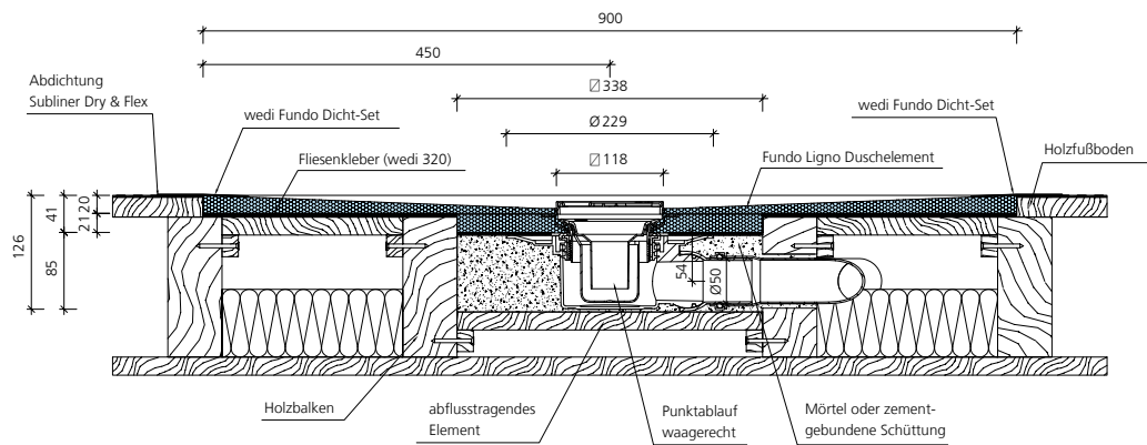
wedi Fundo Punktablauf waagerecht, DN 50, in Holzbalkendecke
