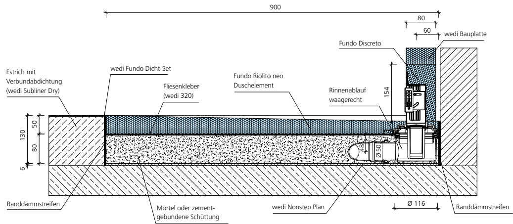
Fundo Discreto, Wandablauf, DN 50, Estrichfußboden
