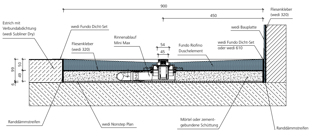
wedi Fundo Rinnenablauf Mini Max, DN 40, Estrichfußboden
