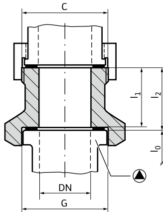
Maßzeichnung
