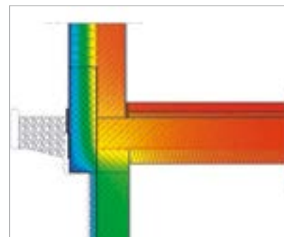
Silka XL auf Kellerdecke über unbeheiztem Keller mit Silka Therm Kimmstein am Wandkopf
