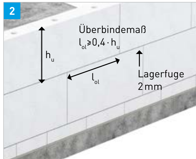
Überbindemaß
