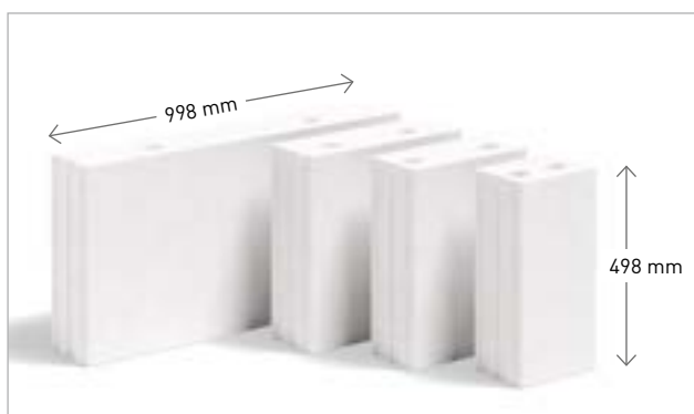
Silka XL-Regel- und Passelemente, Höhe 498 mm
