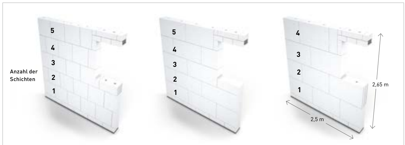
Die Abbildungen zeigen den Vergleich eines Wandausschnittes/Schichtenaufbaus mit Fensteröffnung aus Silka XL L x H = 498 x 498 mm (links), L x H = 998 x 498 mm (Mitte) und L x H = 998 x 623 mm (rechts) bei einer üblichen Geschosshöhe.
