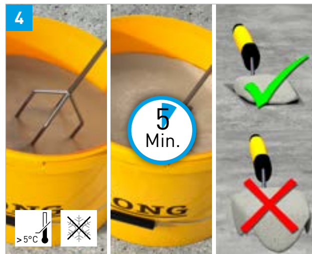
Silka Secure Dünnbettmörtel anmischen (Reifezeit beachten)
