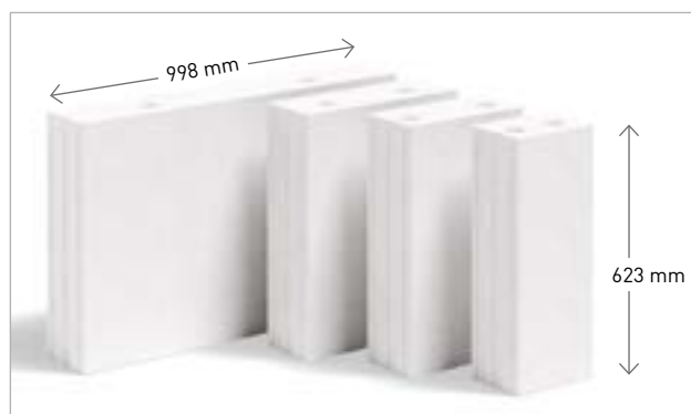
Silka XL-Regel- und Passelemente, Höhe 623 mm
