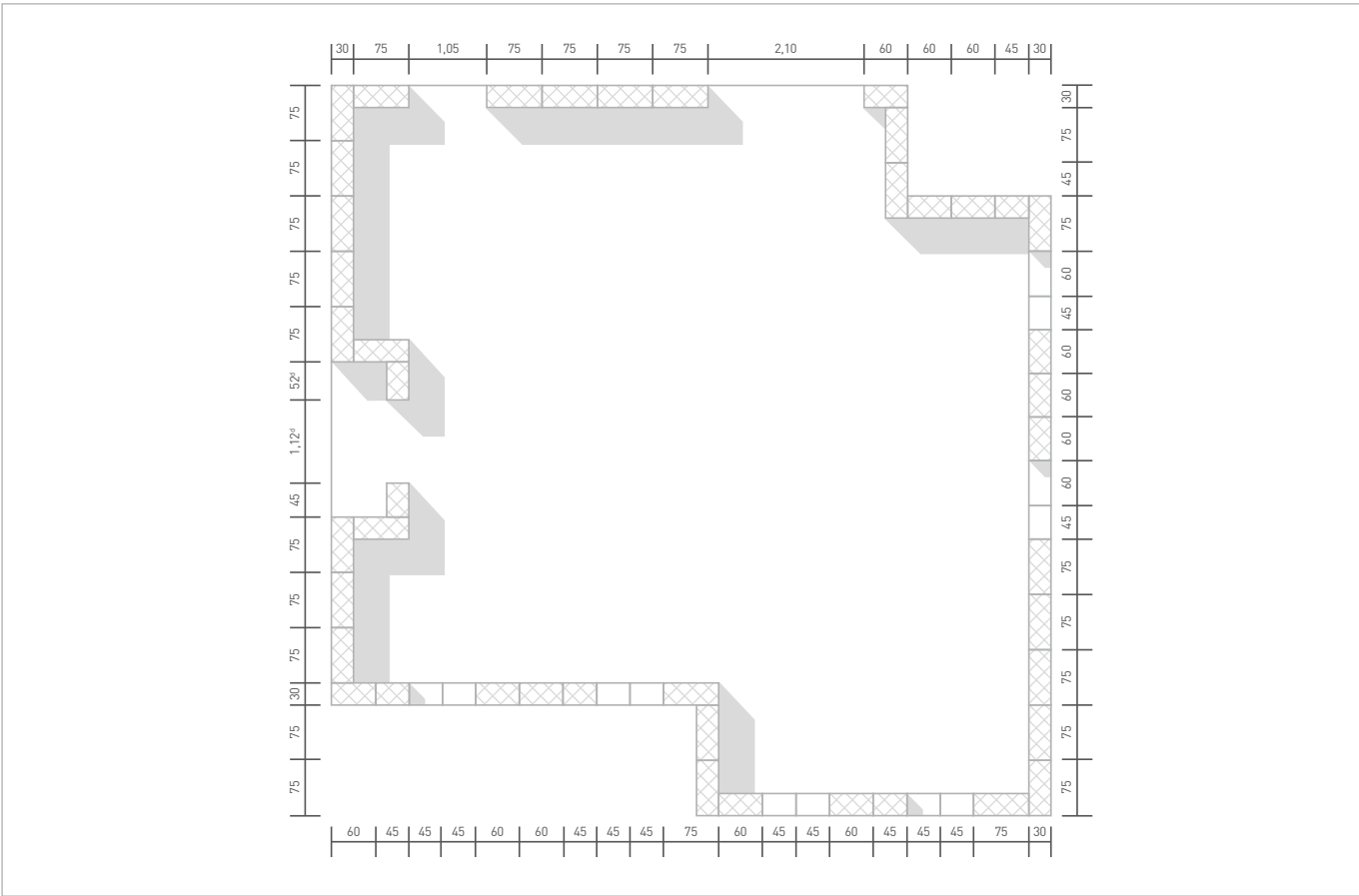
Beispiel einer Grundrissplanung im 7,5 cm Raster
