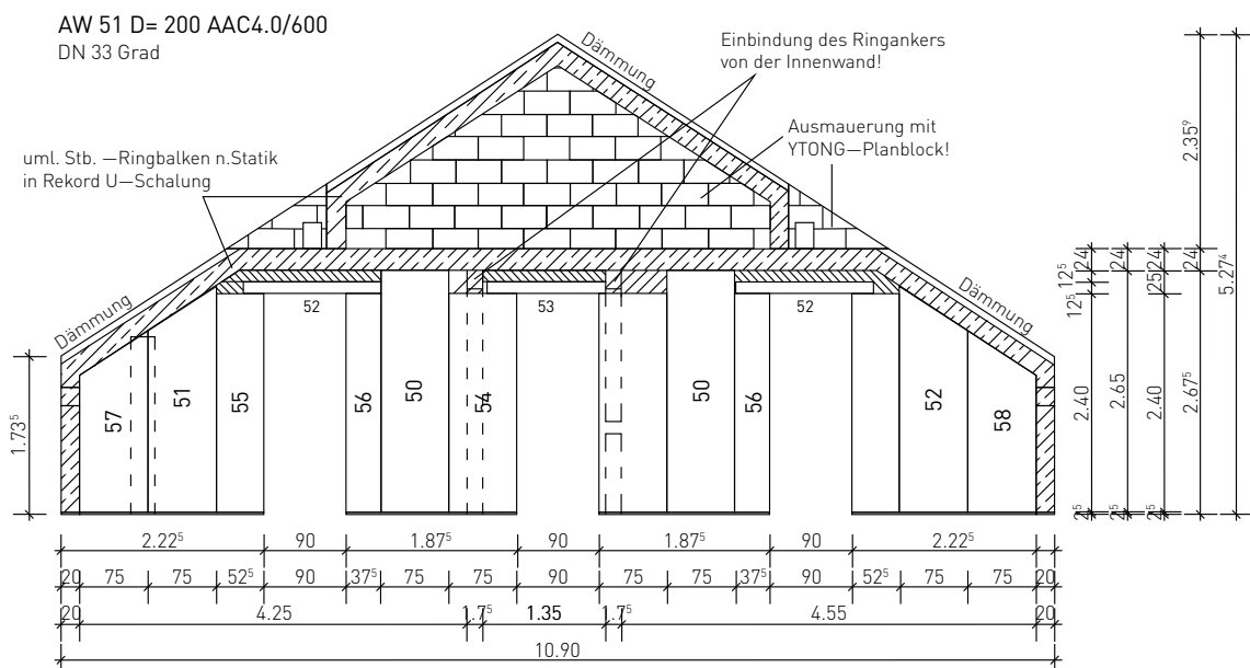
Ausführung mit liegend versetzten Systemwandelementen
