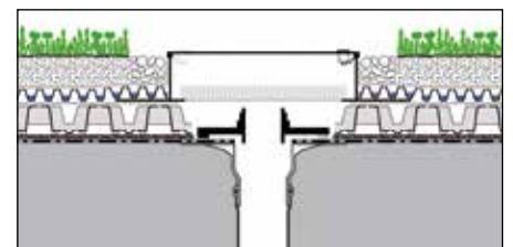
Retentionsdrossel RD 48 zum Einbau über Flachdachabläufen mit Schraubflansch
