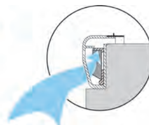
Luftmengenregler geschlossen
