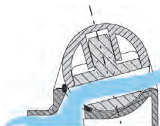
Drehverschluss geöffnet
