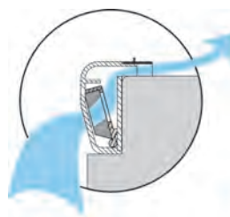
Luftmengenregler geöffnet
