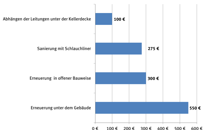
Abbildung 2: Kosten für Sanierungsmaßnahmen je Meter (Beispiele)
