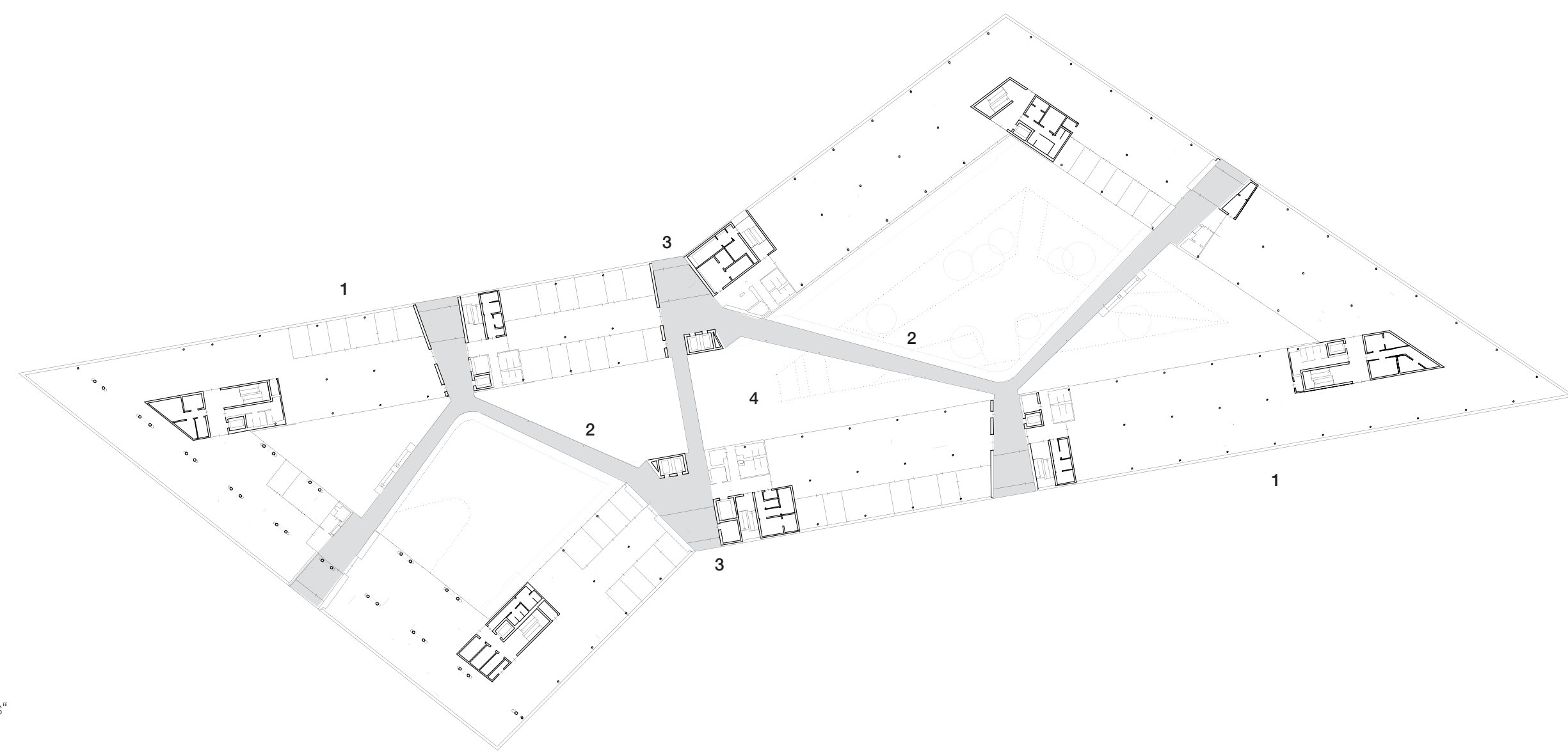
Grundriss 4.OG 1 Flexible Bürolächen 2 Verbindungsstege "Laces" 3 Office Lounge 4 Lufträume
